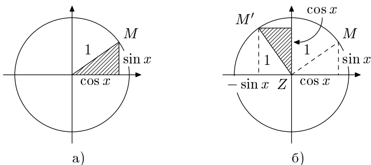
Рис. 9.1. Точка M соответствует числу x , точка M' соответствует числу x + \pi/2 .
