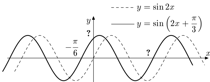
Рис. 11.8. y = \sin(2x + \pi/3) .
