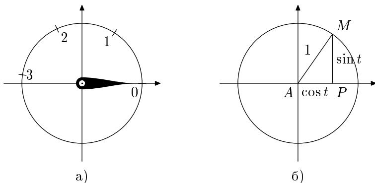
Рис. 5.2. Часы и тригонометрия.
