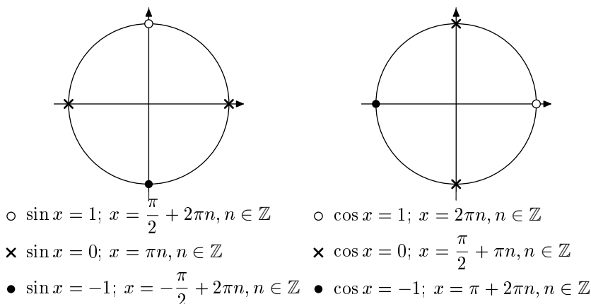
Рис. 10.2. Простейшие уравнения: систематизация.
