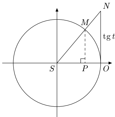
Рис. 6.5. Ось тангенсов. Точка M соответствует числу t
