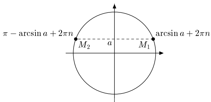
Рис. 10.5. \sin x = a .
