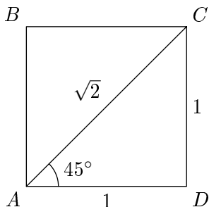
Рис. 3.2. Функции угла 45^\circ .
