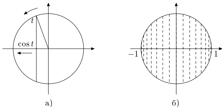
Рис. 5.3. Как меняется косинус.
