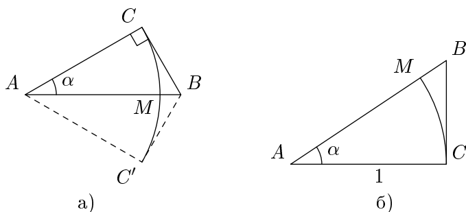
Рис. 2.3. \operatorname{tg} \alpha > \alpha .
