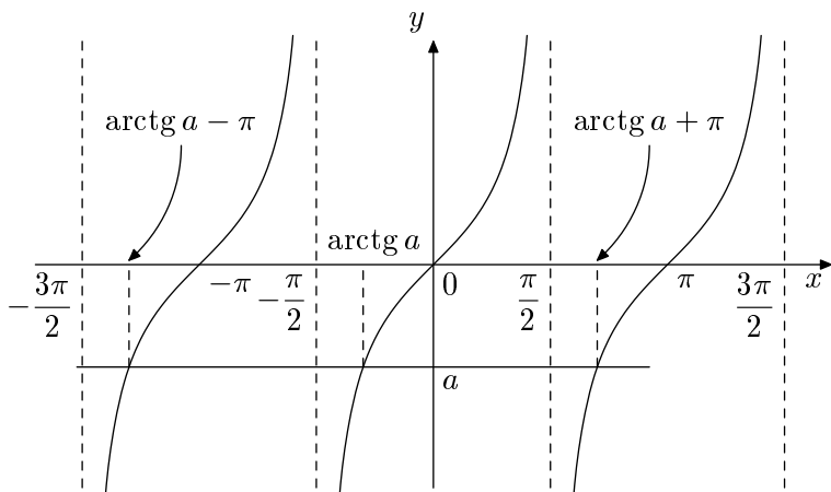
Рис. 12.2. y = \operatorname{tg} x .
