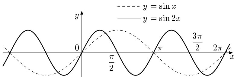
Рис. 11.7. y = \sin 2x .
