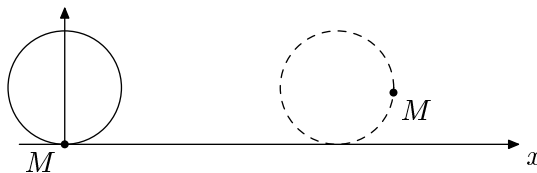
Рис. 6.4. Точка M движется по циклоиде.
