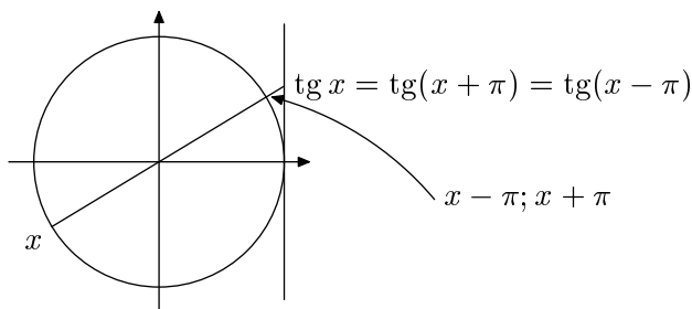
Рис. 8.1. Период тангенса и котангенса.
