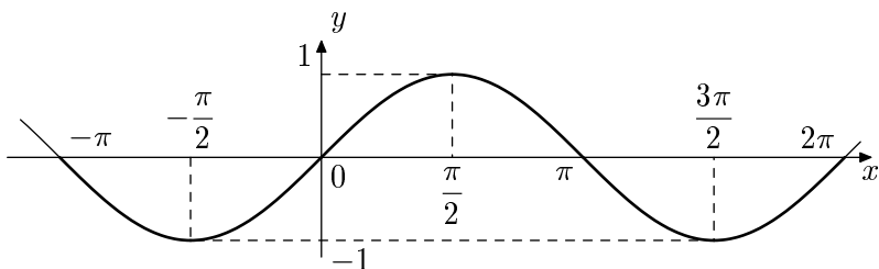
Рис. 11.4. y = \sin x .
