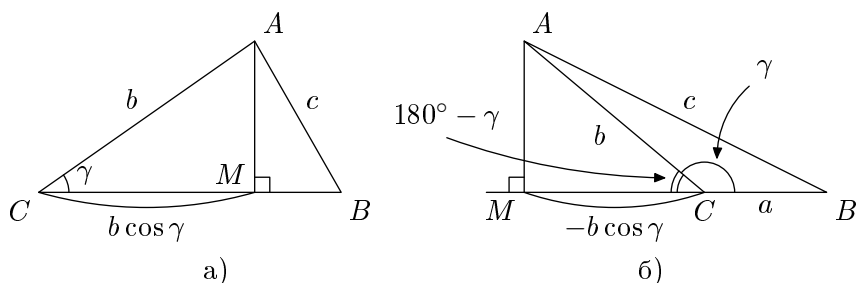
Рис. 14.1. На рис. 14.1а имеем a = BC .
