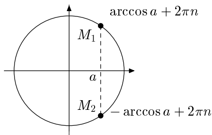
Рис. 10.7. \cos x = a .
