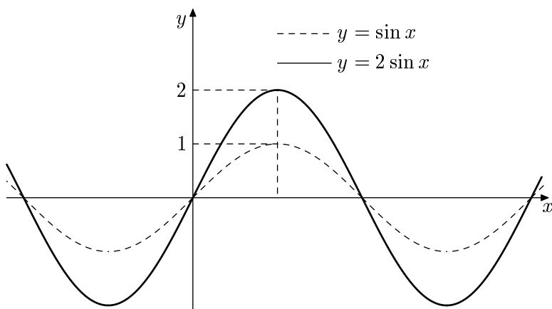
Рис. 11.6. y = 2 \sin x .
