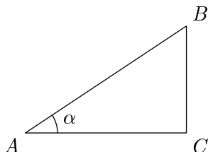
Рис. 1.3. \sin \alpha = BC/AB .
