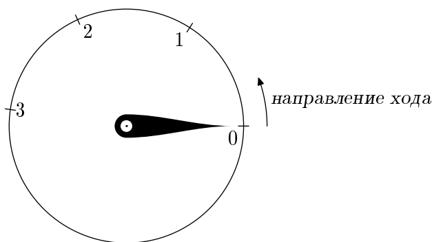
Рис. 5.1. Часы фирмы «Тригонометрия». Длина каждой из трех дуг равна 1.
