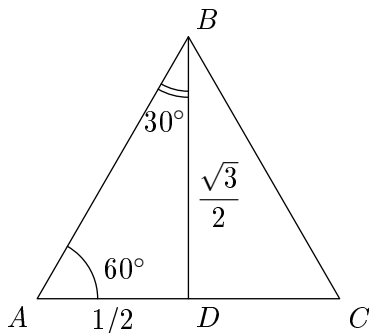
Рис. 3.3. Углы 30^\circ и 60^\circ .
