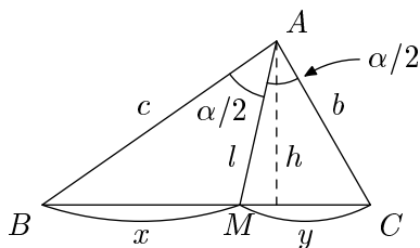
Рис. 15.5. Теорема о биссектрисе.
