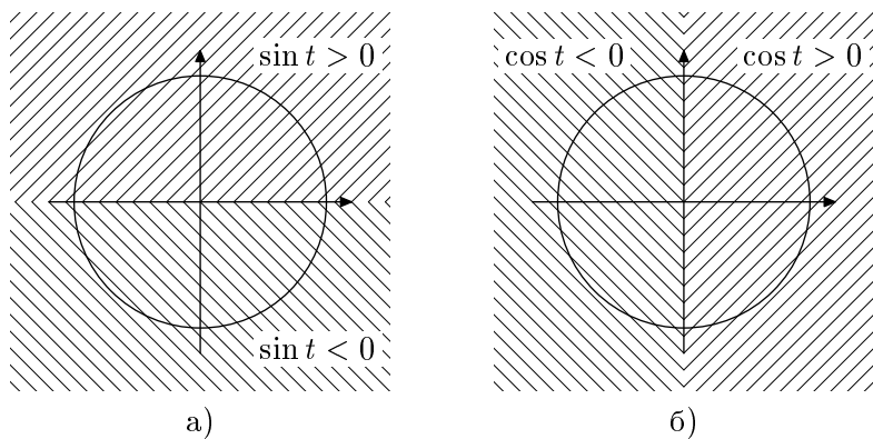
Рис. 6.6. Знаки синуса и косинуса.
