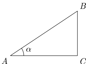
Рис. 3.1. \cos \alpha = AC/AB .
